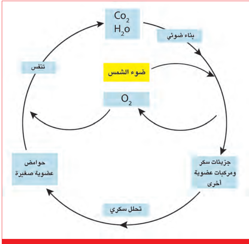
شكل (2-1). الاتجاهات الرئيسية لدورة الكربون
