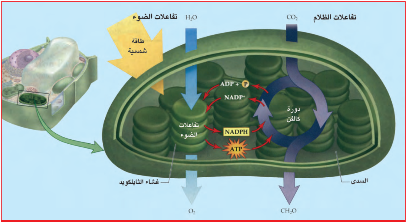
شكل (1-2) مخطط عام لعملية البناء الضوئي (تفاعلات الضوء وتفاعلات الظلام أو ما يعرف بدورة كالفن).
